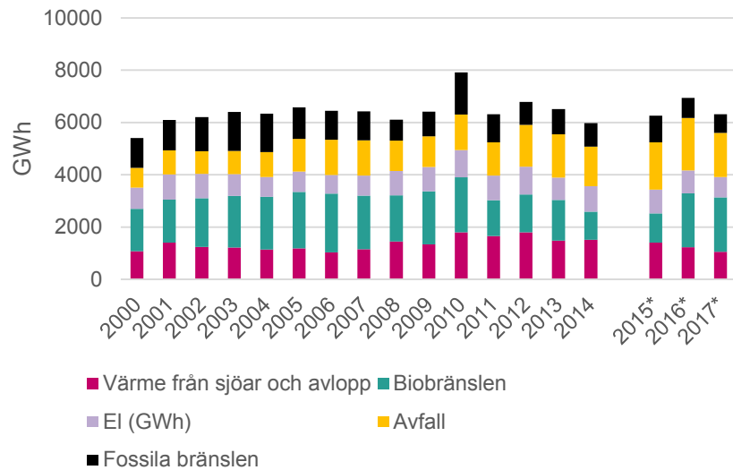
Figur 4 Insatta bränslen och energier (ej normalårskorrigerade värden) i fjärrvärmesystem för produktionsanläggningar inom Stockholms stads geografiska gräns 2000-2014, *2015-2017 avser produktionsanläggningar för det regionala fjärrvärmenätet
