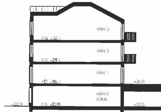
PRINCIPSEKTION
