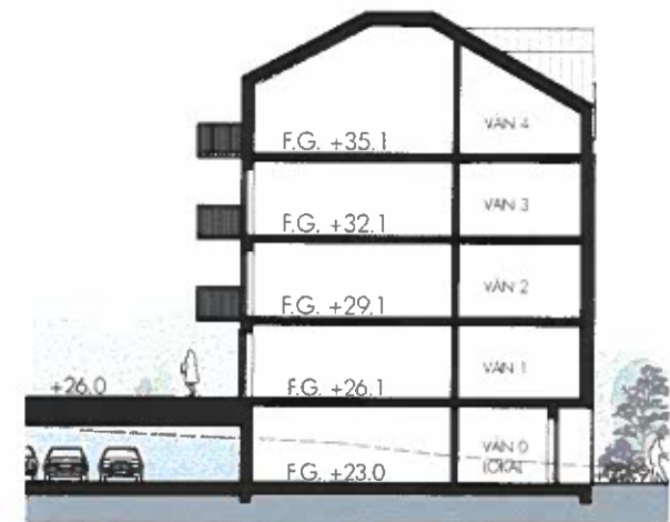
PRINCIPSEKTION
