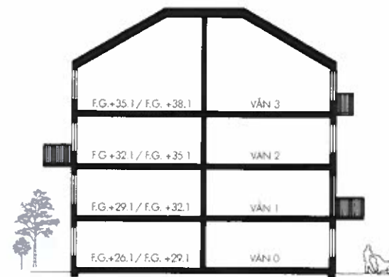
PRINCIPSEKTION
