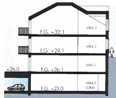
PRINCIPSEKTION
