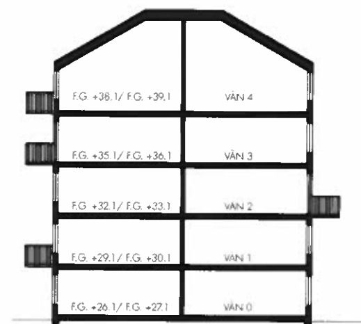
PRINCIPSEKTION
