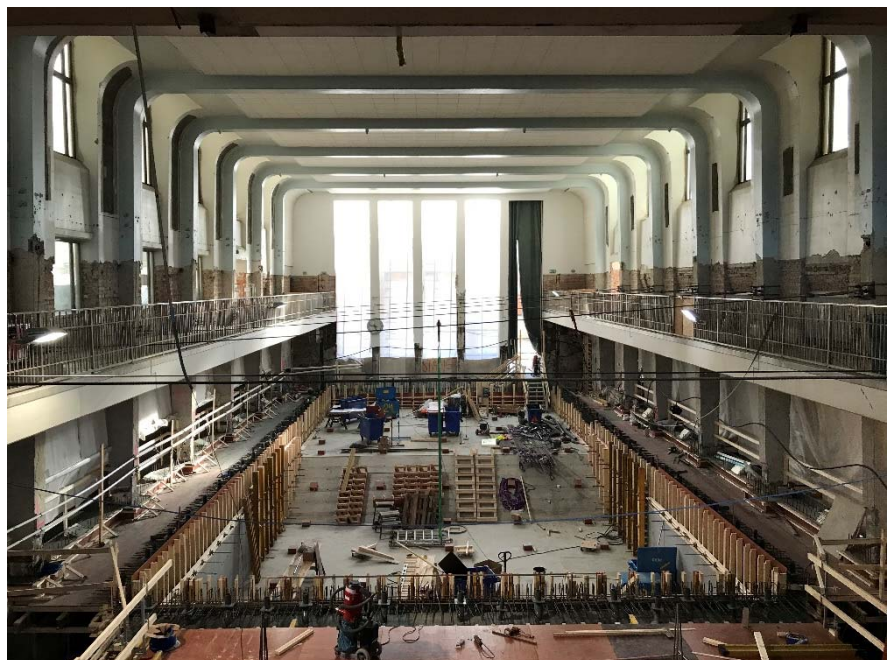
Bassänggjutning pågår.
