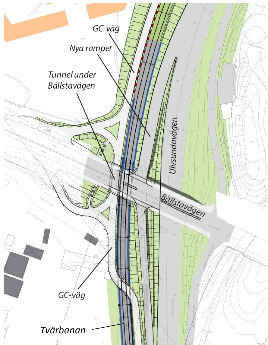
Bild 2. Utformning av nya Solvallakopplet samt gång- och cykelramper. (Bild från SL, Tvärbana Norr Kistagrenen)
