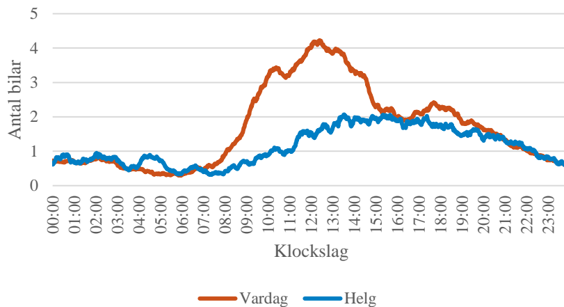
Figur 10. Antalet bilar som snabbladdar samtidigt under en genomsnittlig vardag och helgdag år 2018.
