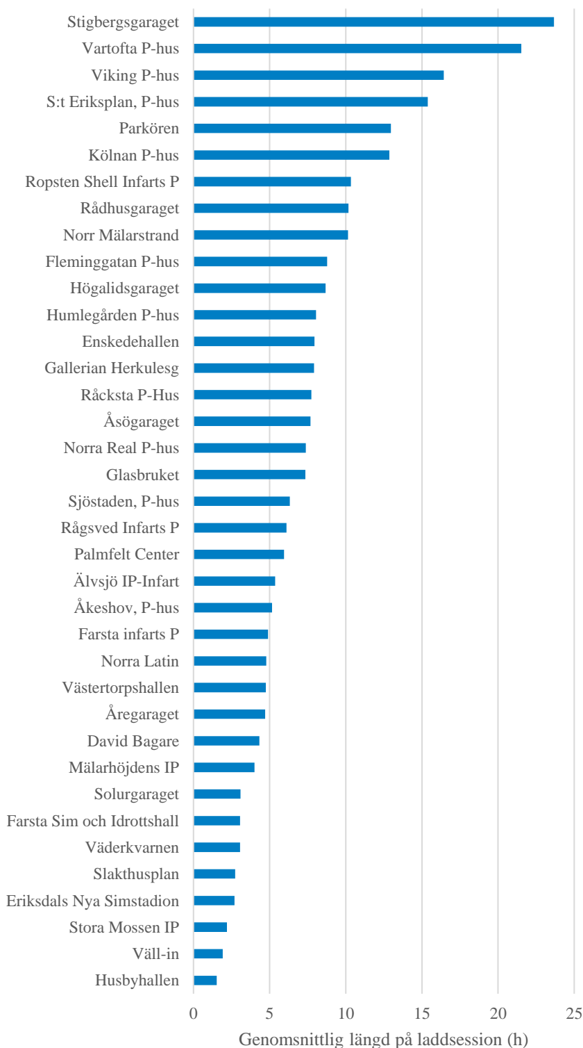
Figur 19. Genomsnittliga laddtider för Stockholm Parkerings parkeringsanläggningar under år 2018.
