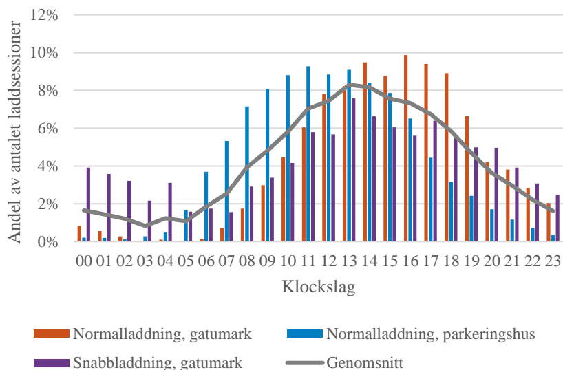
Figur 8. Andelen laddsessioner år 2018 som påbörjats vid ett visst klockslag under dygnet på helgen för respektive laddningskategori.
