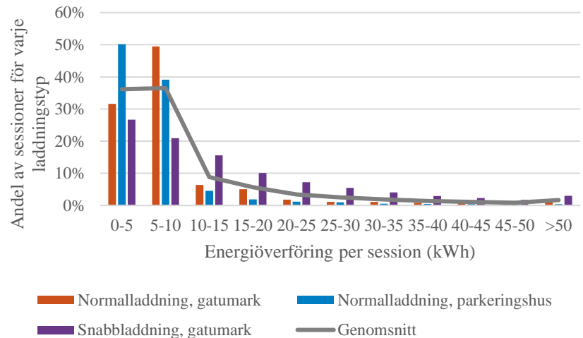
Figur 23. Andelen sessioner för respektive laddningstyp år 2018 fördelat på överförd energimängd.
