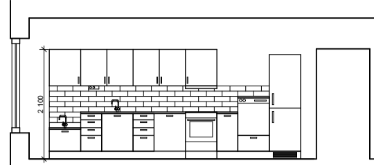
ELEVATION KÖK I TORG
