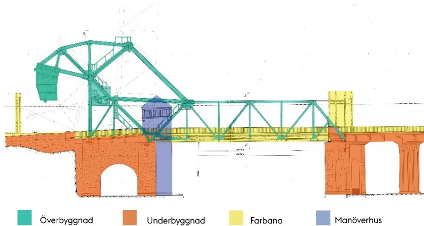
Figur 3. Norra Damviksbrons huvudsakliga delar (Stockholms stads stadsmuseum 2018).
