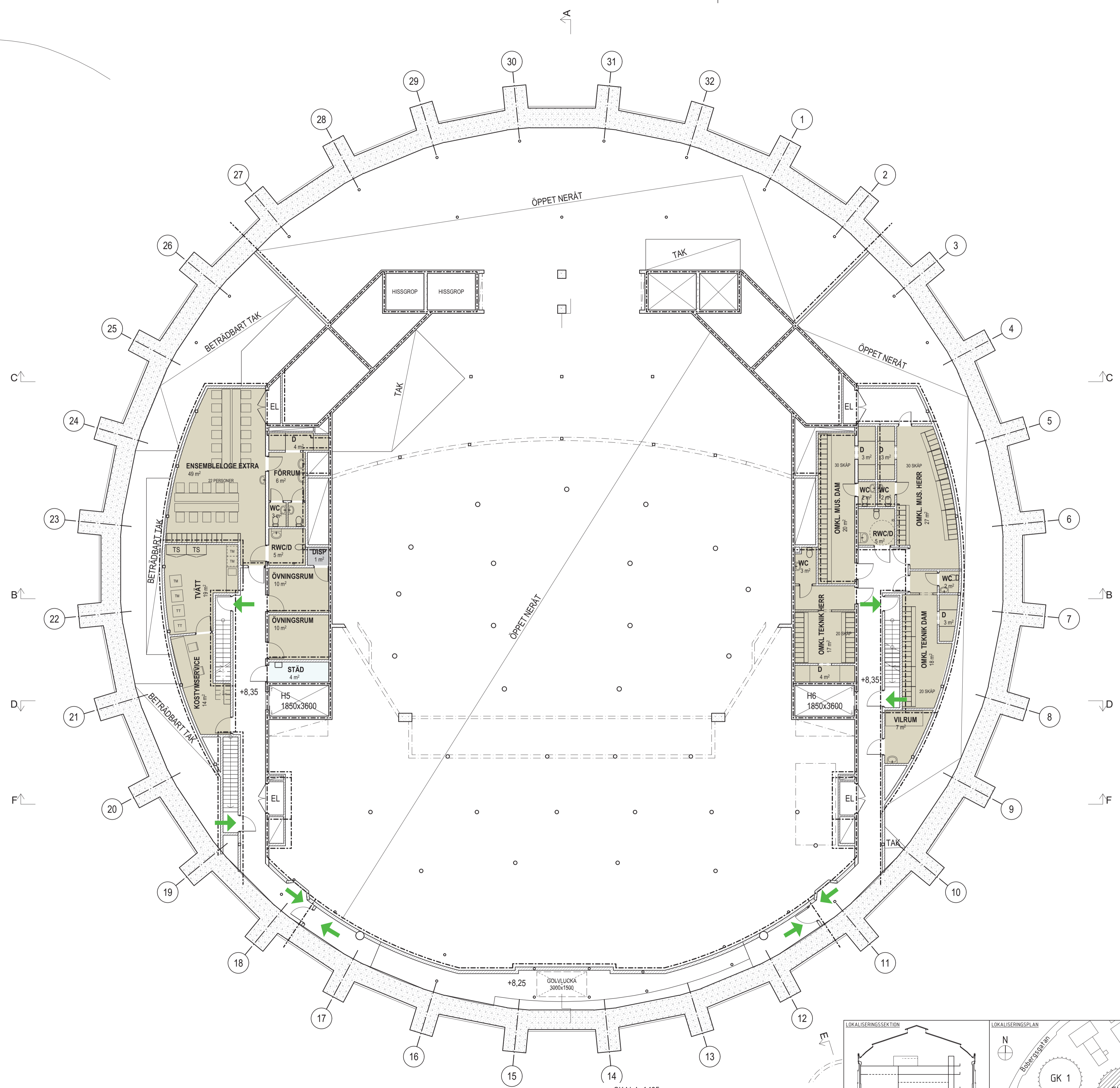
Plan 2 - Källare Skala 1:125
