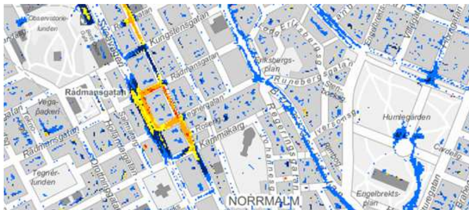
Resultat från Stockholms skyfallmodell, maximalt vattendjup vid 100-årsregn
