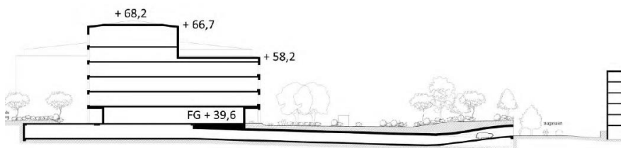
Sektion av skola och garage i nord-sydlig riktning. Bildkälla: Max Arkitekter
