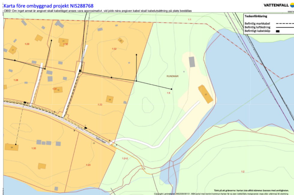
Figur 2 visar dragning av befintlig luftburen ledning
