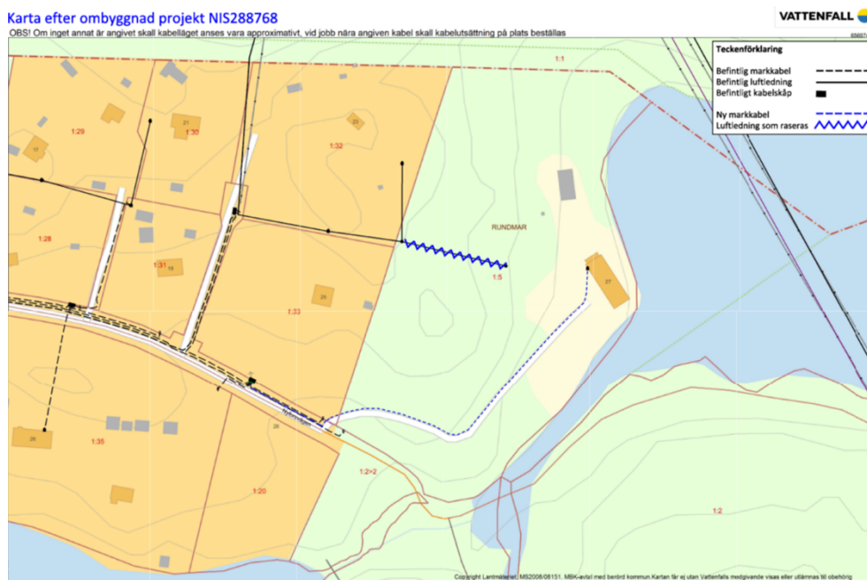
Figur 3 befintlig luftdragen ledning rives, blå punktlinje visar sträckning för ny markledning
