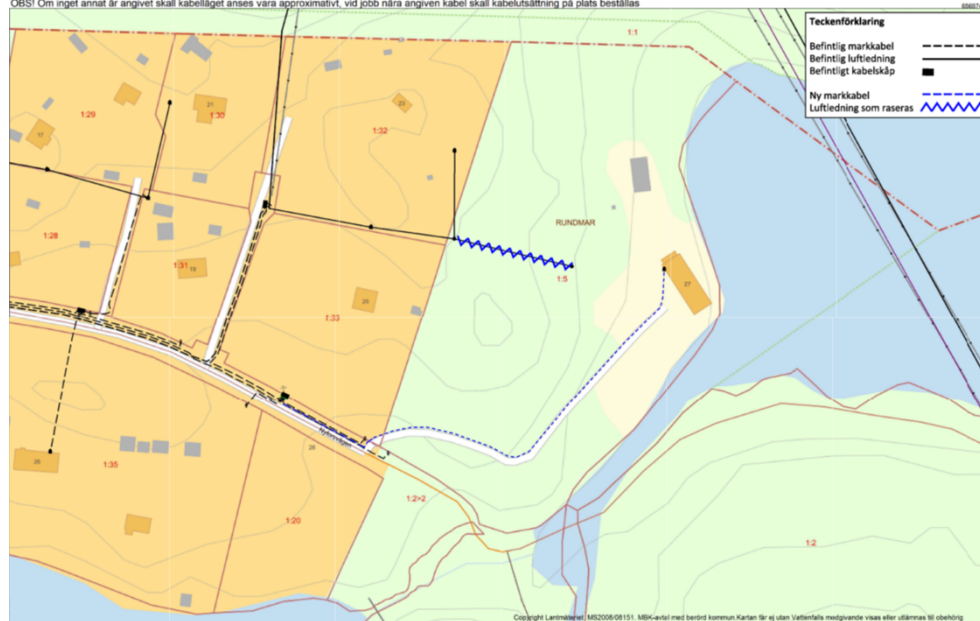
Figur 3 befintlig luftdragen ledning rives, blå punktlinje visar sträckning för ny markledning
