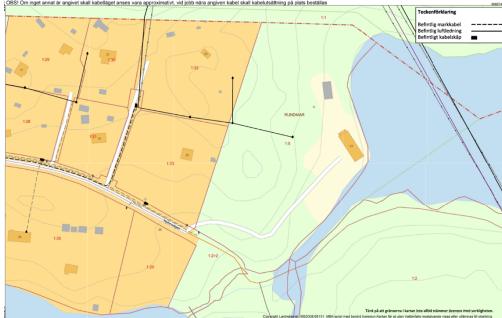
Figur 2 visar dragning av befintlig luftburen ledning
