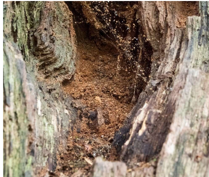
Figur 22. Många vedlevande insekter är beroende av mulm, det vill säga det lösa material som ansamlas inuti ihåliga och oftast gamla träd. Vid avsaknad av hålträd och mulm kan uppsättning av mulmholkar vara ett värdefullt komplement för att gynna de vedlevande insekterna. Foto: Mattias Bovin.
