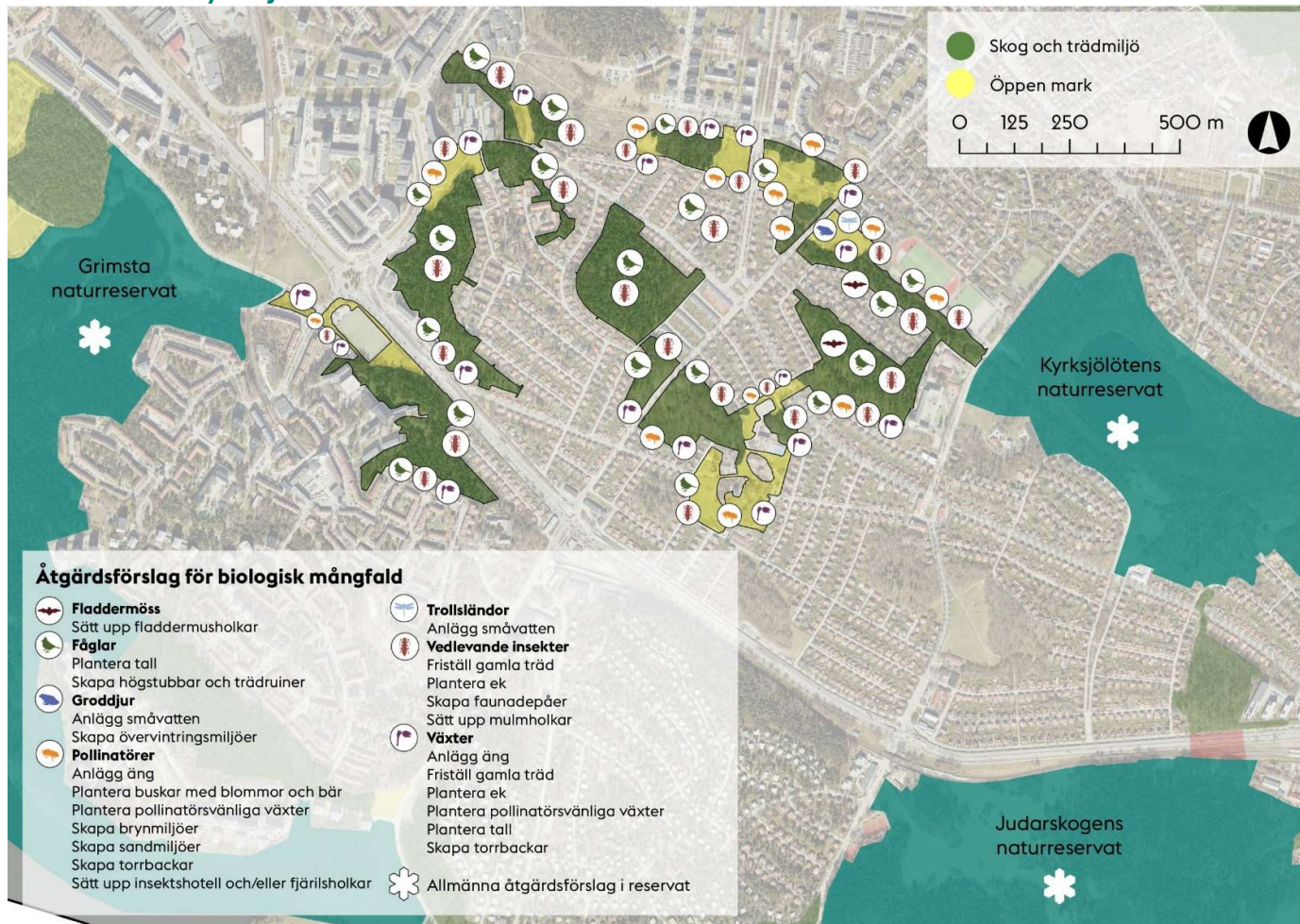
Figur 19. Åtgärdsförslag för biologisk mångfald i Grimsta-Kyrksjölötenstråket. Använd matrisen i figur 3 för att tolka kartan.
