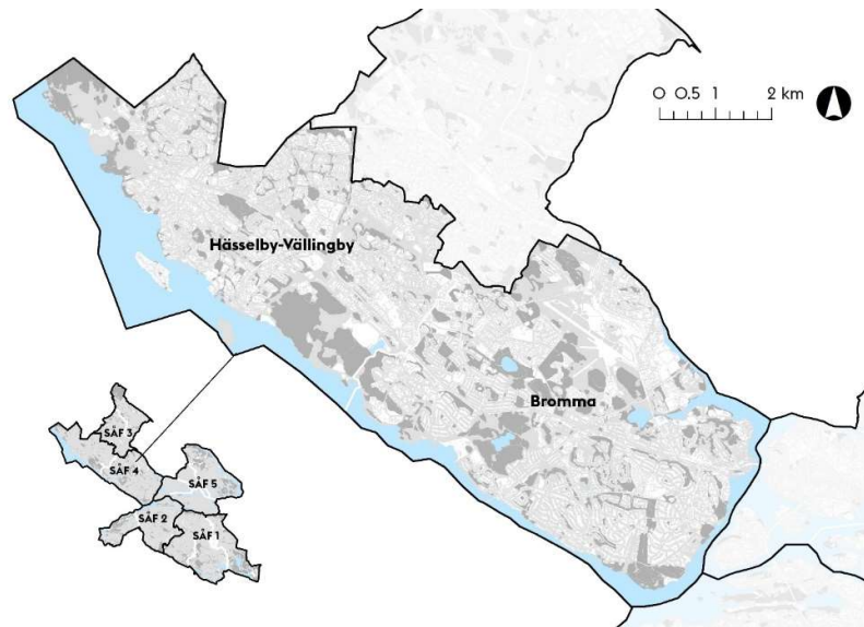
Figur 1. Projektområde för stadsdelsvist åtgärdsförslag för biologisk mångfald i Hässelby-Vällingby och Bromma.
