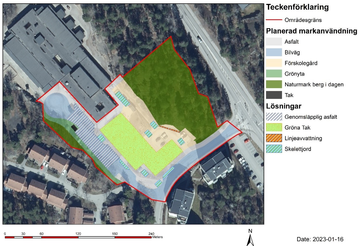
Figur 14: Skalenliga lösningar utifrån planerad höjdsättning samt illustrationsplan, linjeavvattnings placering är ungefärlig. Bakgrundskarta © Lantmäteriet.
