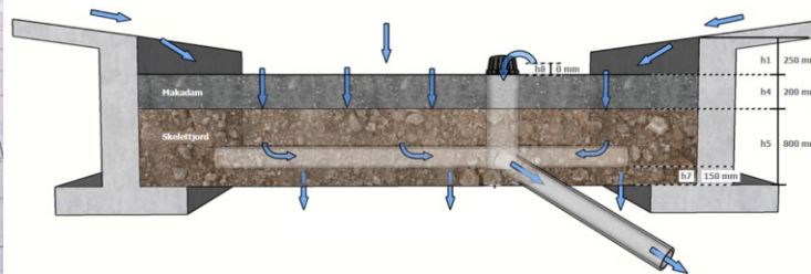
Figur 11: Exempelbilder på skelettjord samt principskiss över skelettjord med fördröjningsvolym ovanpå (Stormtac 2022).
