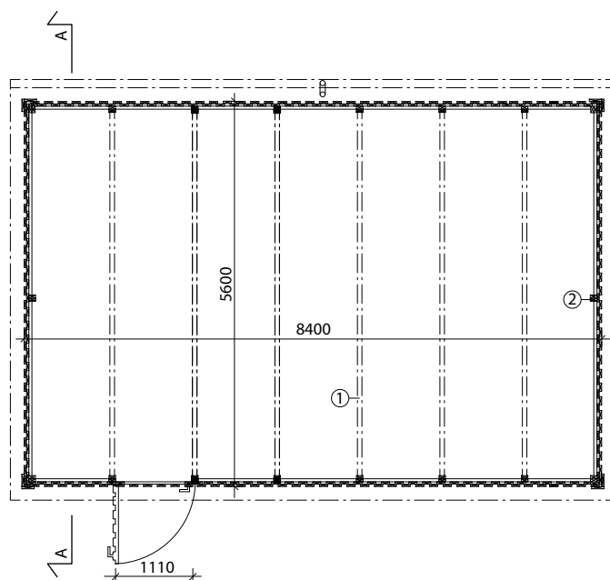
PLAN 1:100
