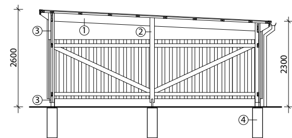
SEKTION A-A 1:100
