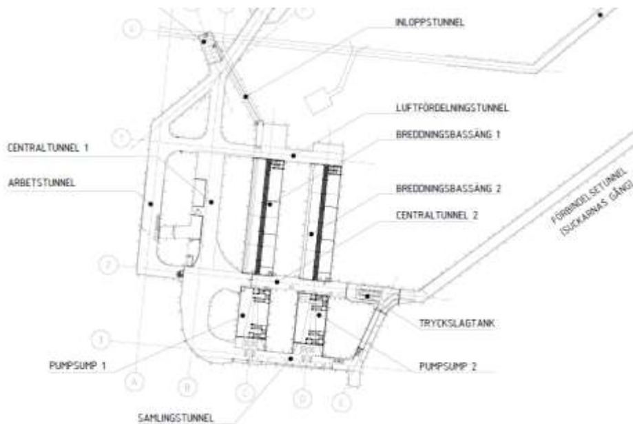
Figur 2 - Översiktsskiss över AP Knösen plan 0.
