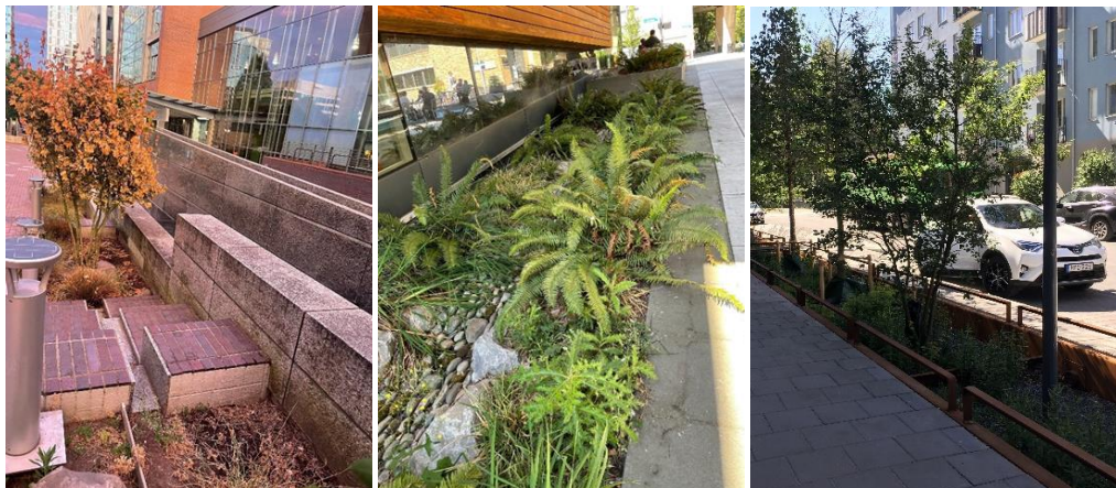
Bild 5, 6 och 7. Bilder på nedsänkta växtbäddar i Portland (5 och 6) och Norra Djurgårdsstaden (7). Foto från Portland av Sophie Jutterström, 2022
