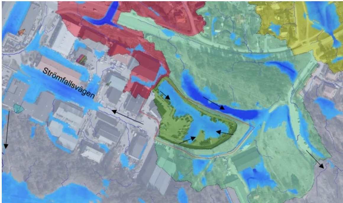
Figur 14. Bild som visar avrinning vid skyfall, samt instängda områden, utan hänsyn till dagvattenledningsnätet. Svarta pilar visar flödesriktning. Utredningsområdet är markerat med röd linje (Bjerkäng, 2024-04-09)
