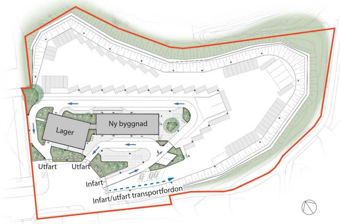
Figur 5. Illustrationsplan som visar föreslagen utformning. Körslingar är markerade med blå pilar. In- och utfart för transportfordon är markerad med blå, streckad linje. Röd linje markerar föreslagen plangräns. (PE Teknik & Arkitektur, 2024-03-14)
