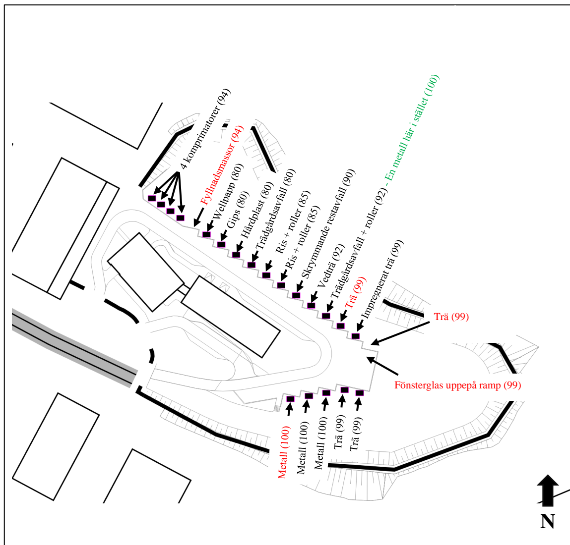
Figur 8. Fiktivt utökad scenario där ändringarna är markerade i rött. För det ytterligare utökade fiktiva scenariot tillkommer förändringen som har markerats i grönt.
