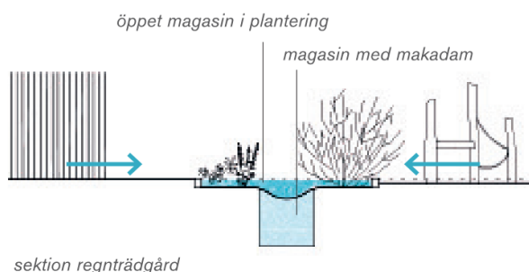
Figur 4 Sektion regnträdgård.
