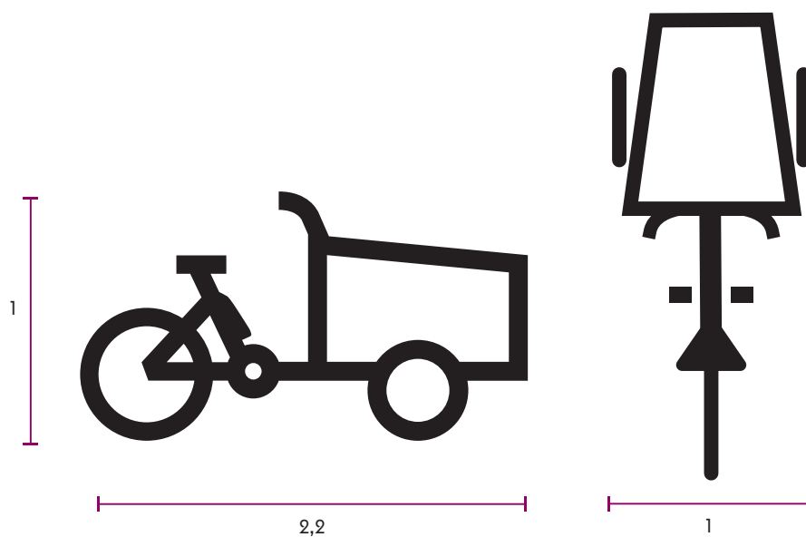
Figur 2. Bredd-, längd- och höjdmått för en utrymmeskrävande cykel.
