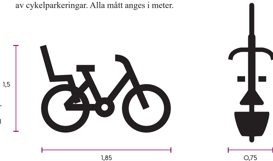
Figur 1. Bredd-, längd- och höjdmått för en cykel med barnstol.
