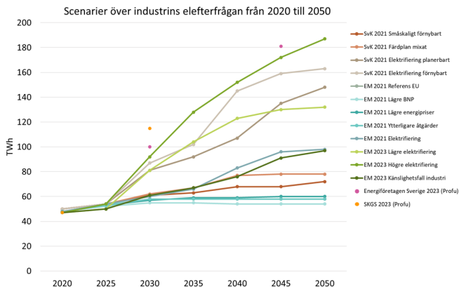
Figur 1. Utvecklingen av industrins elefterfrågan (TWWh) enligt olika scenarier från Svenska Kraftnät (SvK), Energimyndigheten (EM), Energiföretagen Sverige samt SKGS från 2020 fram till 2050. Som framgår sträcker sig spannet från dagens elbehov på knappt 50 TWWh till nästan 190 TWWh år 2050 i det mest elintensiva scenariot, dvs. ett utfallsrum på 140 TWWh (motsvarande dagens totala elbehov för alla sektorer i Sverige).
