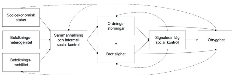
Figur 2. Icke-rekursiv teoretisk modell på områdesnivå av otrygghet. Inspirerad av modeller från Bursik och Grasmick (1993), Hinkle (2009), Hunter (1978), Markowitz et al. (2001) samt Wikström och Dolmén (2001). Hämtad och översatt från Kronkvist (2022).
