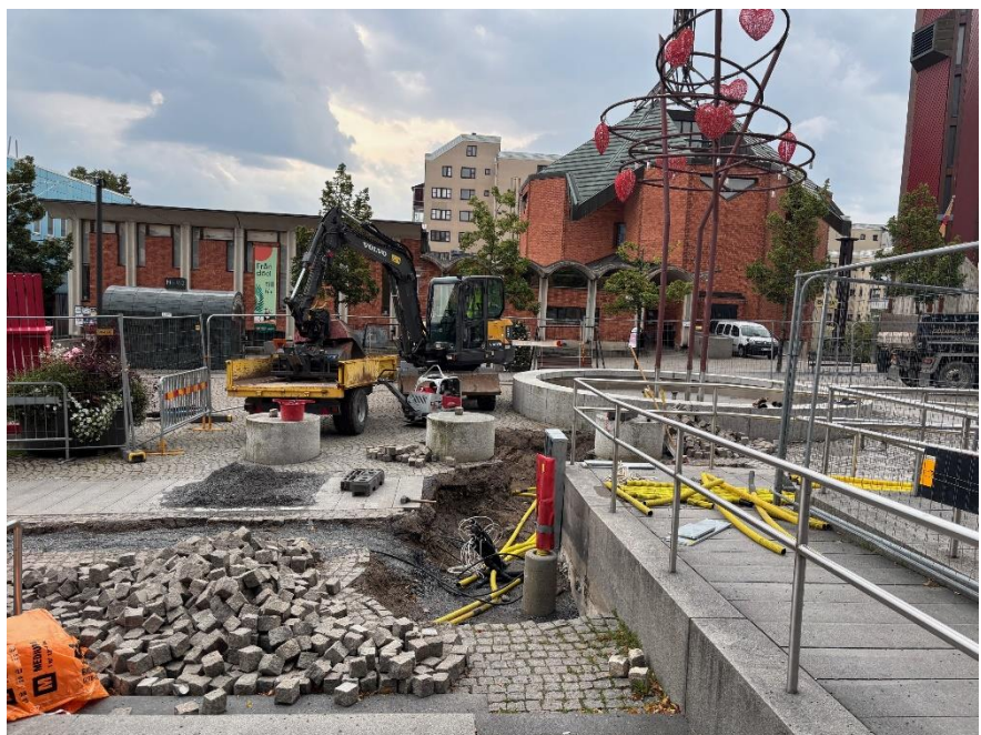
Byggskede belysning
