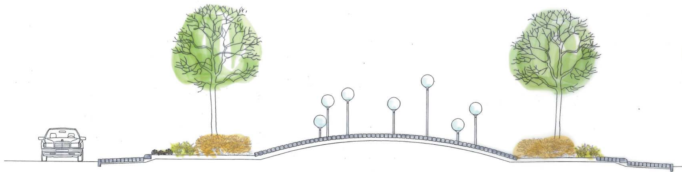
SEKTION A-A SKALA 1:20
