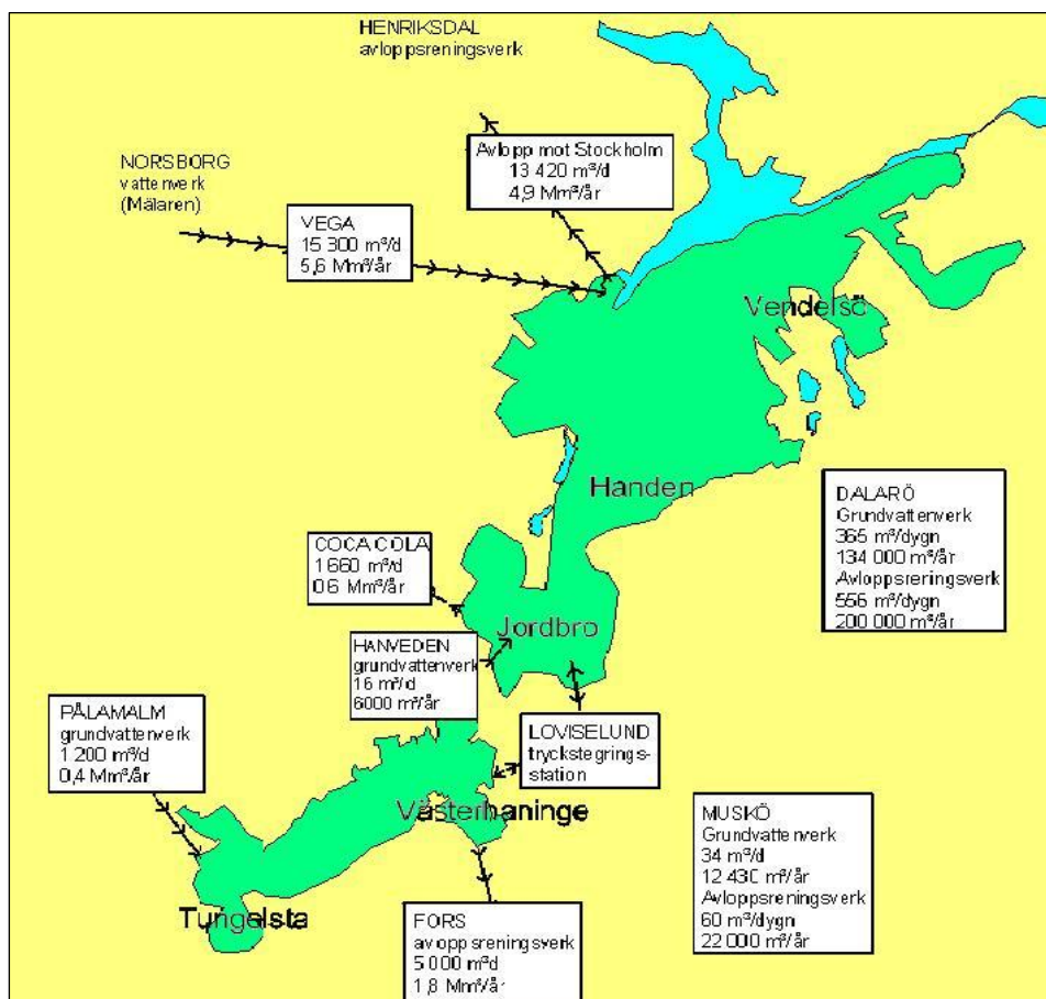
Bild 16: Viktiga komponenter i Haninge kommuns spillvattensystem. GIS-karta: Hans Kristiansson
