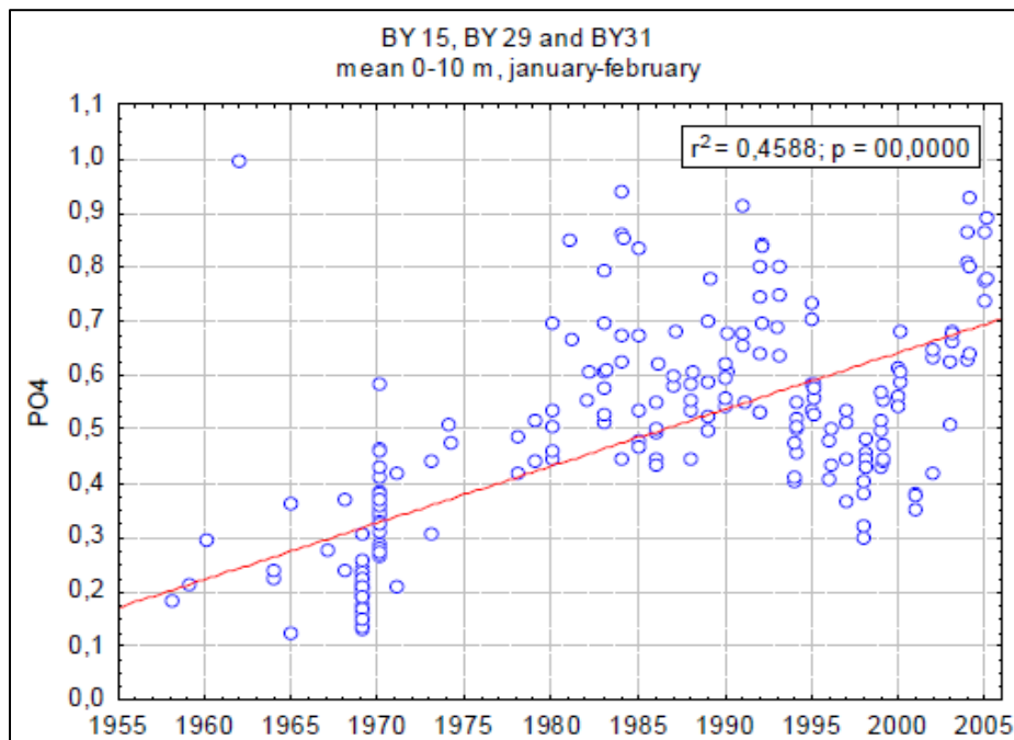
Bild 22: Utvecklingen av halten löst fosfat i Östersjön åren 1955 – 2005. Källa: SMHI
