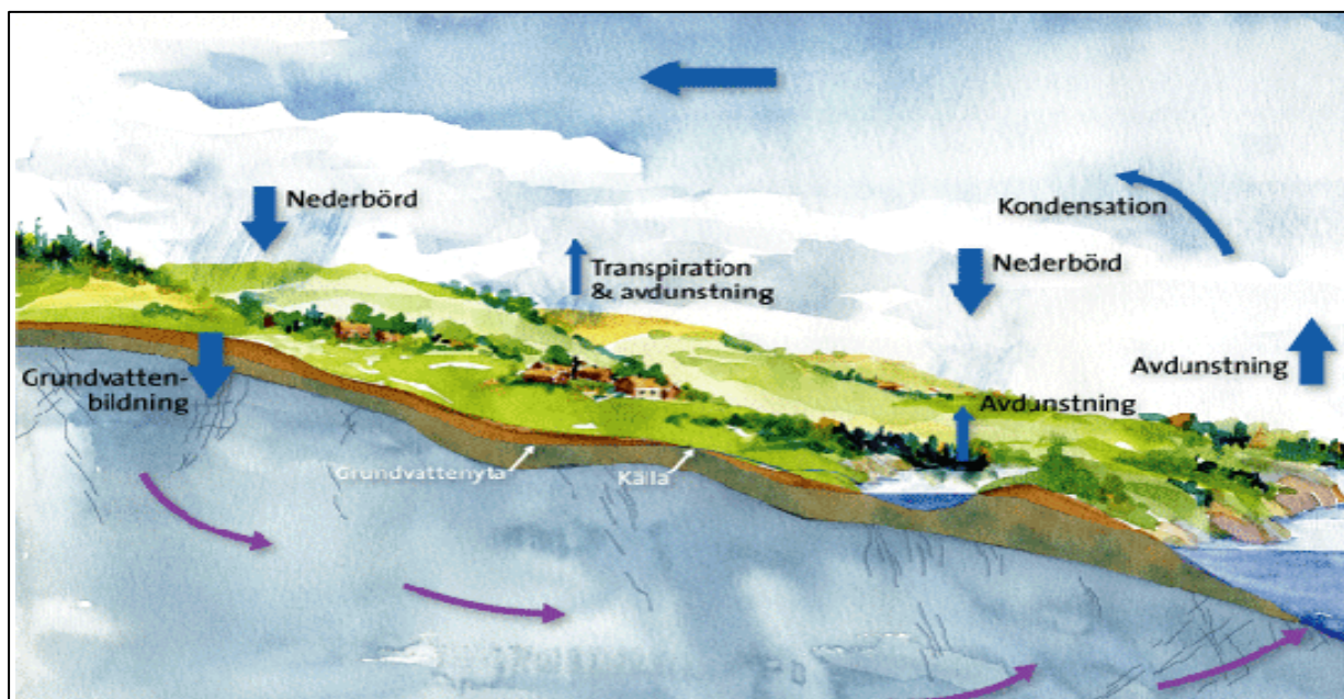
Bild 5: Vattnets kretslopp/den hydrologiska cykeln. Hur grundvatten skapas. Copyright SGU
