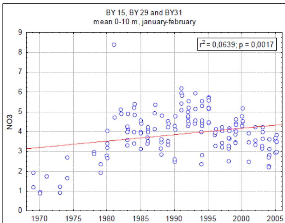
Bild 23: Utvecklingen av halten löst kväve (nitrat) i Östersjön 1970 – 2005.
