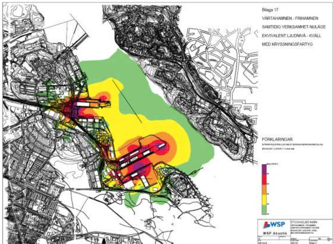
Bullerutbredning, nuläge
