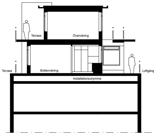
Sektion D-D
