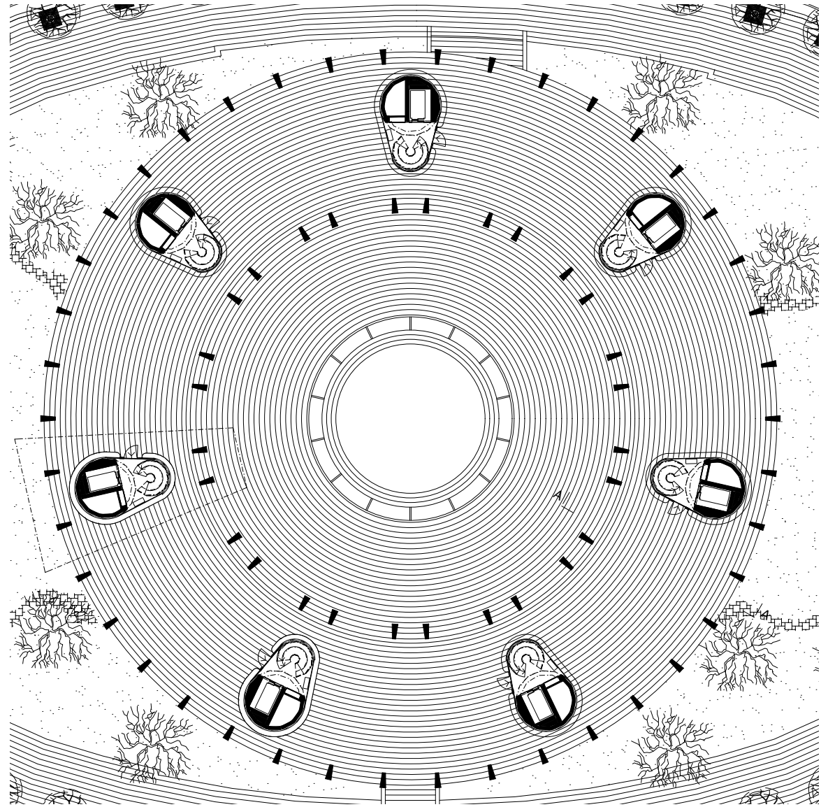
Entréplan skala 1:400
