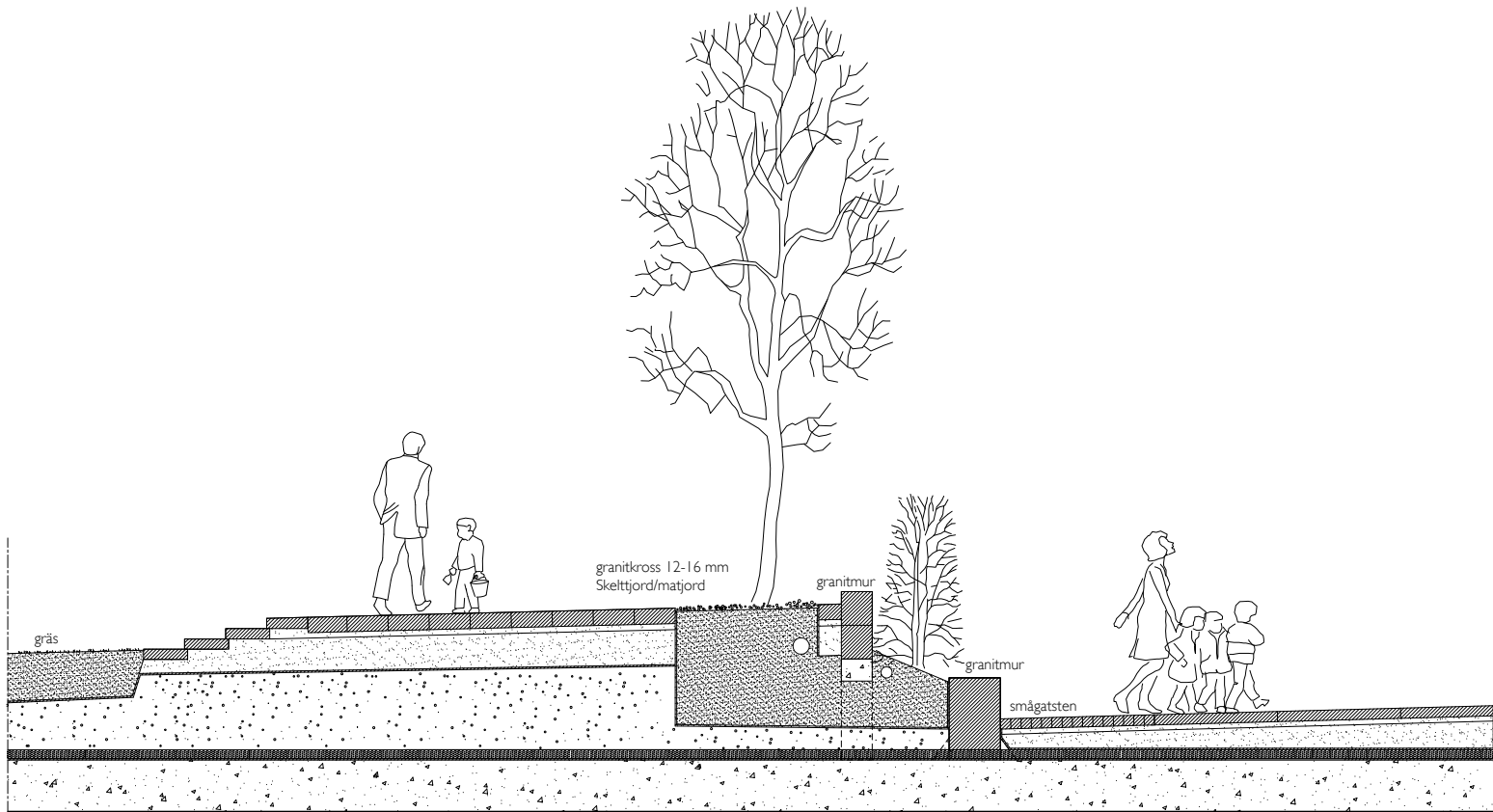
Snitt genom mur
