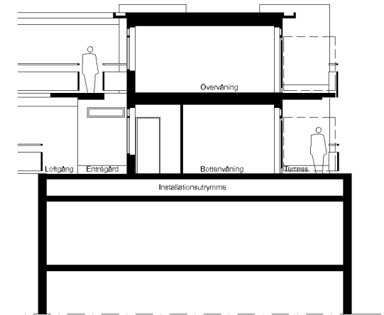
Sektion E-E
