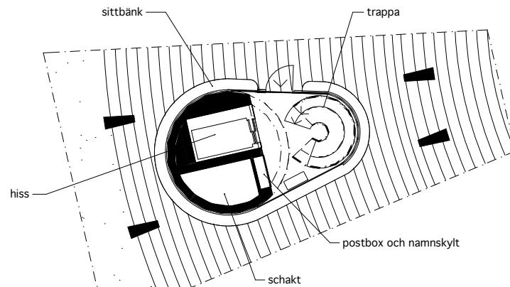
Plan av entréhall skala 1:200
