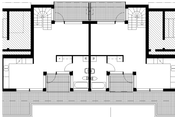
Nedre plan
