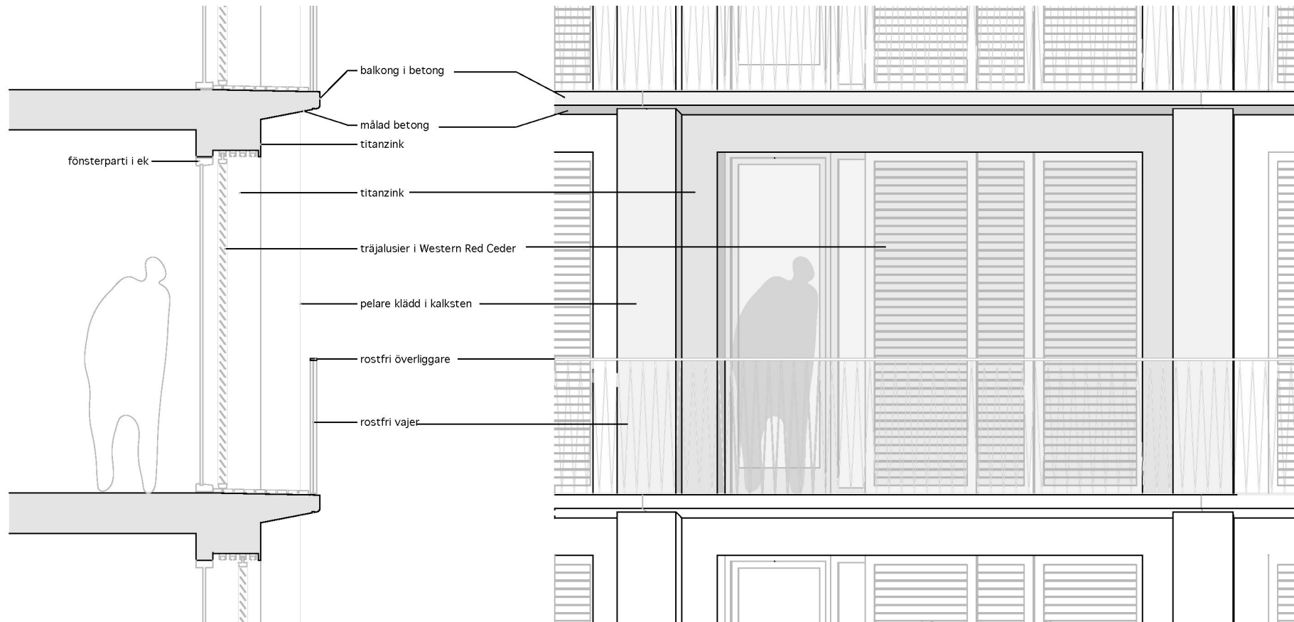
Fasadutsnitt fransk balkong, fönsterparti och jalusier skala 1:50
