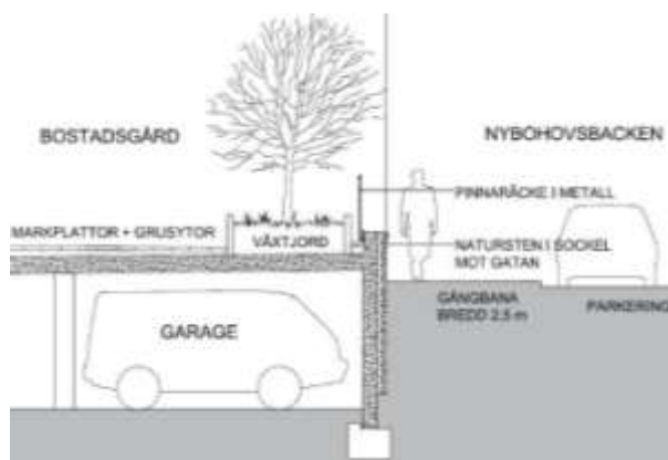
Snitt genom gårdsyta i område A. Stödmur/sockel i natursten, upphöjd växtbädd och underliggande garage
