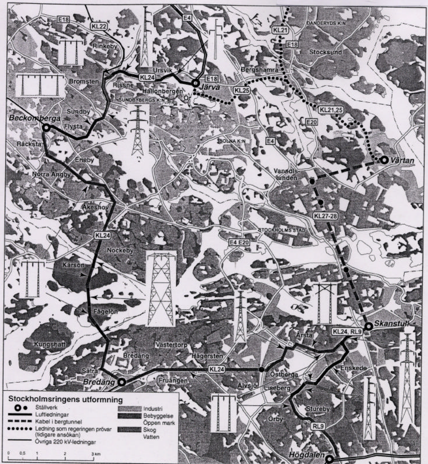
Figur 2 Stockholmsringens utformning med ledningsbeteckningar och de vanligast förekommande stolptyperna.
