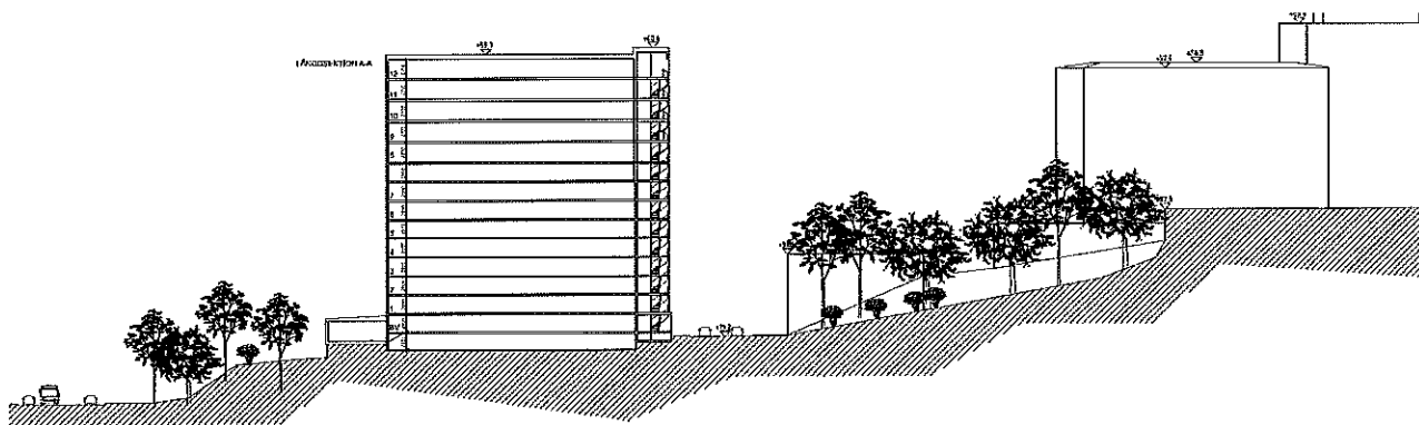
Tvärsektion med befintlig Gärdesbebyggelse till höger bild.
