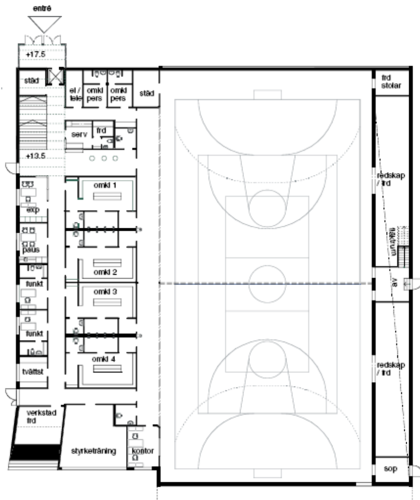
Planskiss Skanstullshallen
