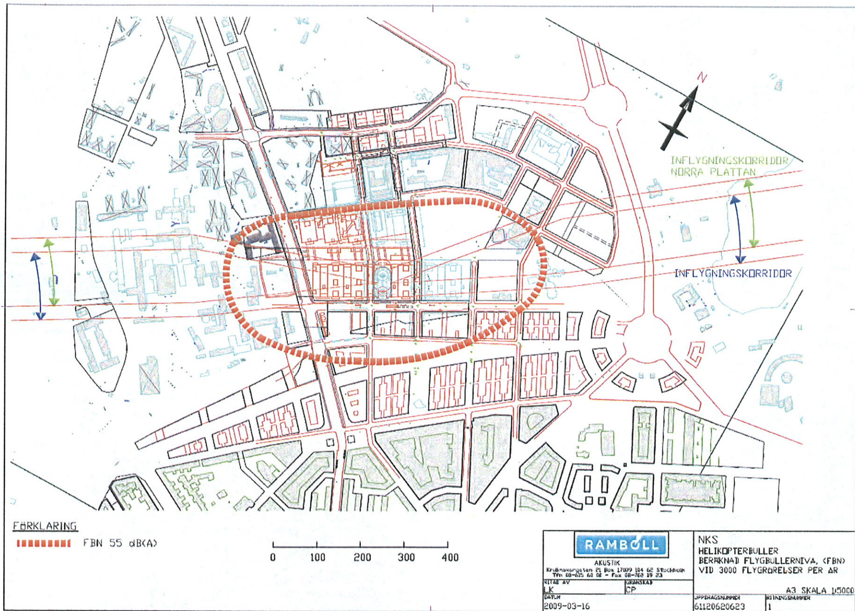
Figur 8 b. Beräknad gräns för 55 dB ekvivalent bullernivå vid start och landning enligt planförslaget. Kvartersstrukturen kan vara inaktuell.
