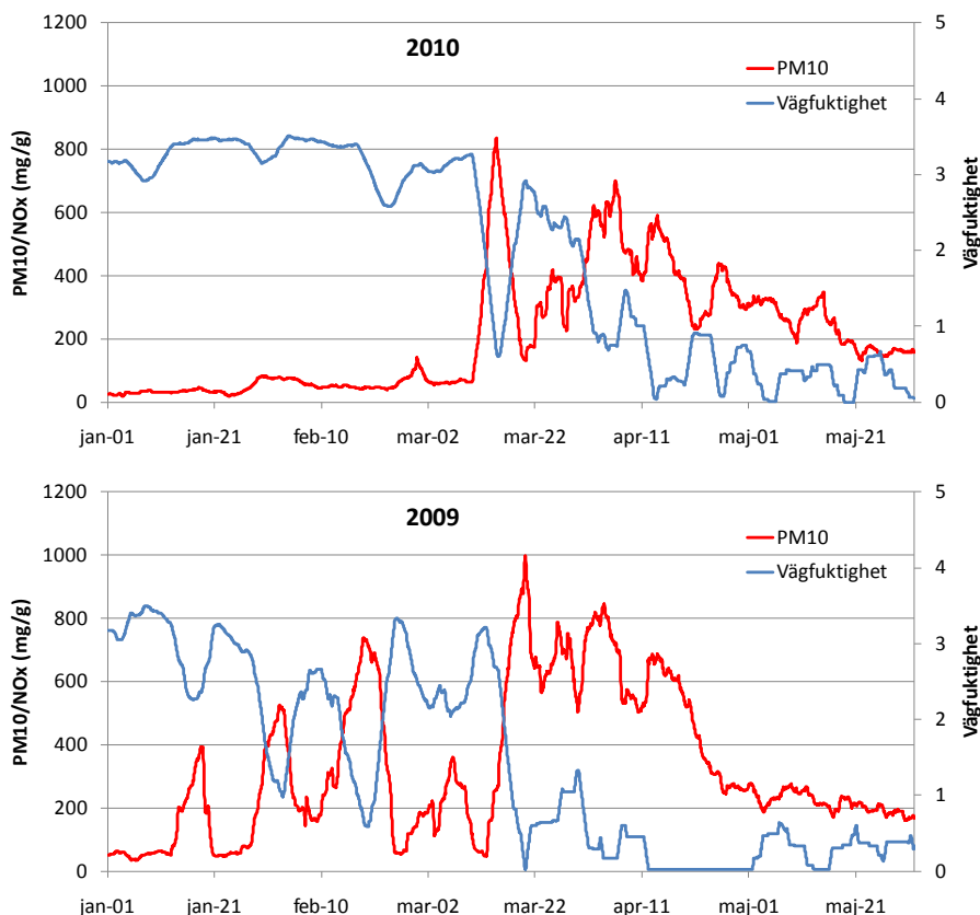
Relationen mellan mängden PM10 per gram NOx från trafiken på Hornsgatan och vägbanans fuktighet (högt värde anger fuktig väg bana). Data är baserade på mätningar av PM10- och NOx-halter på Hornsgatan och Torkel Knutssonsgatan (urban bakgrund) under januari – maj 2010 och 2009.
